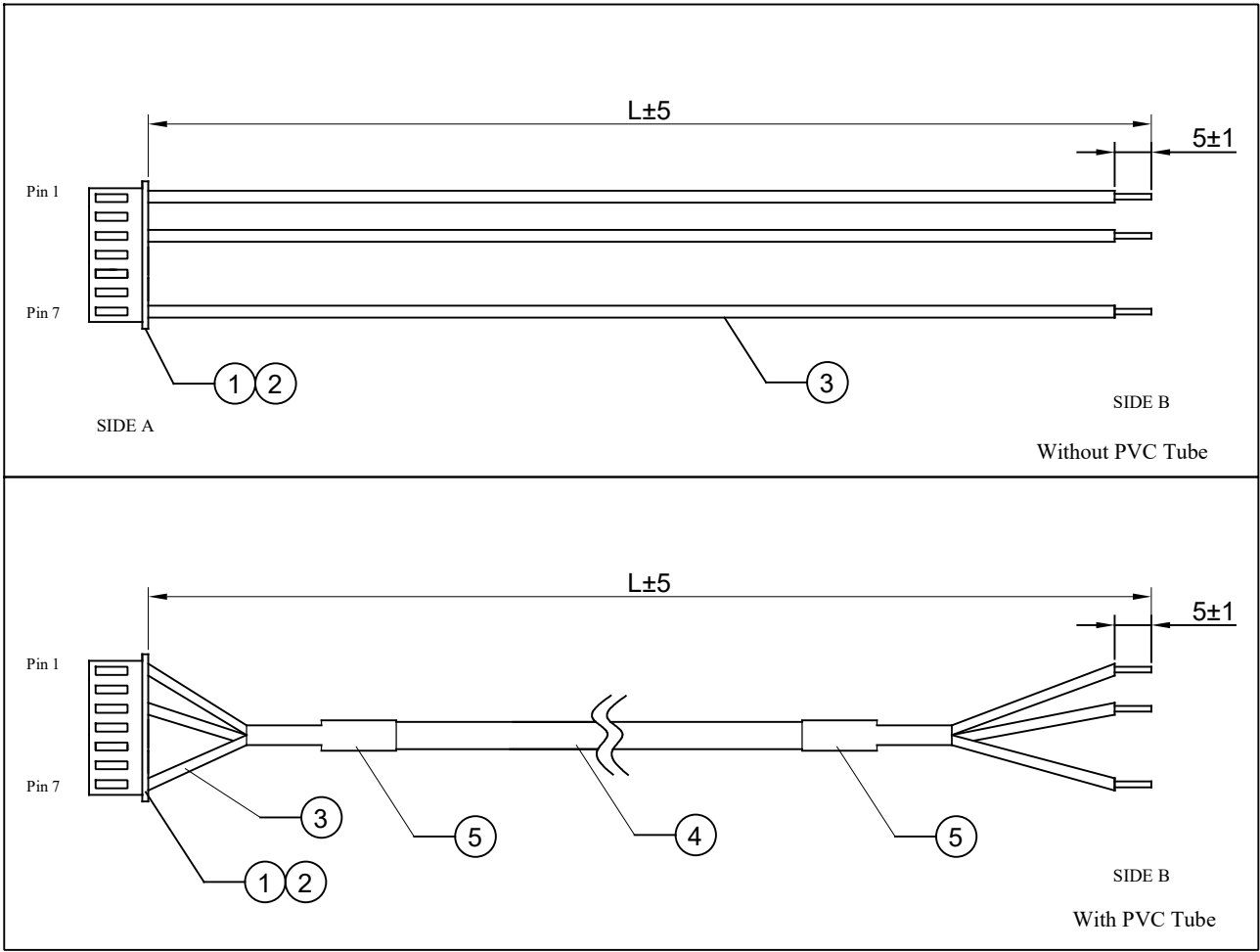
WIRE CHART:
