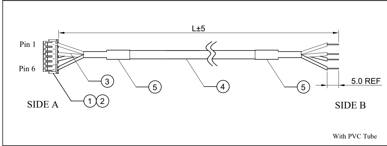
WIRE CHART:
