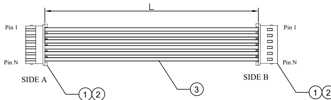
WIRE CHART:
