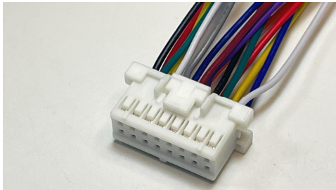
Cable Assembly(Colorful Wires)
